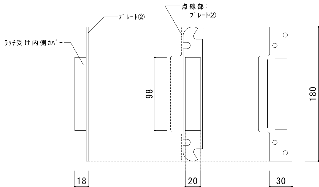
側面図
