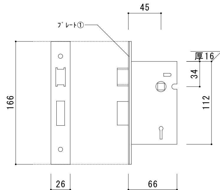
プレート① 正面図 (ホリッシュブラス)
