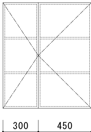
立面図
