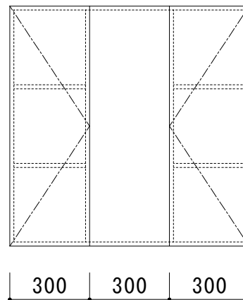
立面図
